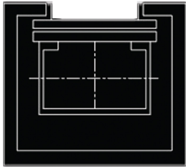
مخطط بئر المصعد
