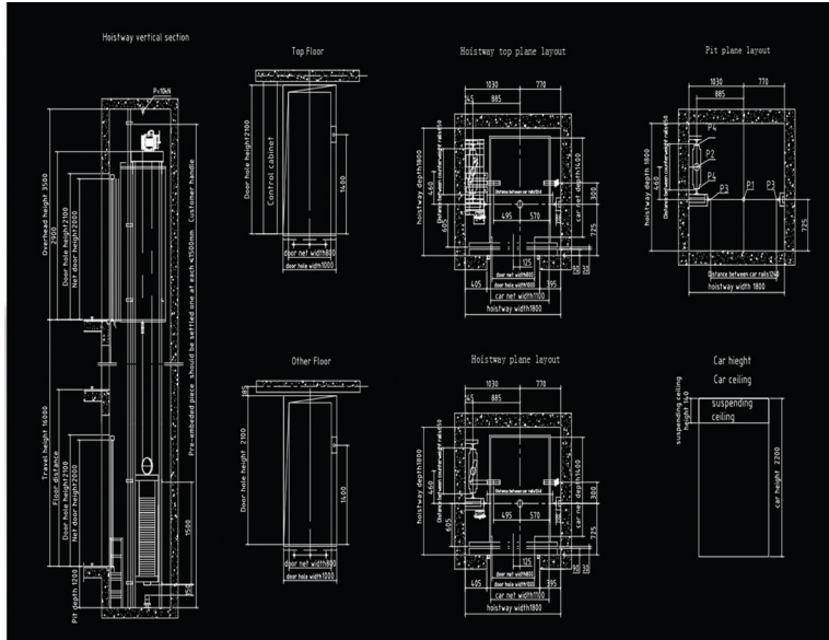
مخطط بئر المصعد Room-less 630
