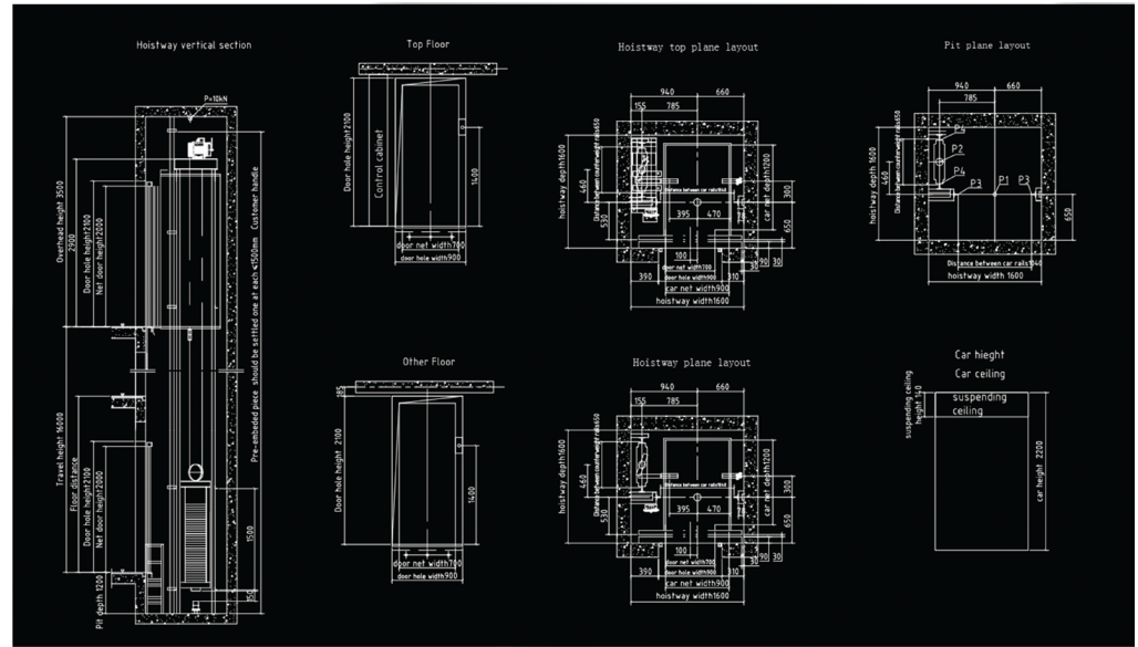
مخطط بئر المصعد Room-less 450
